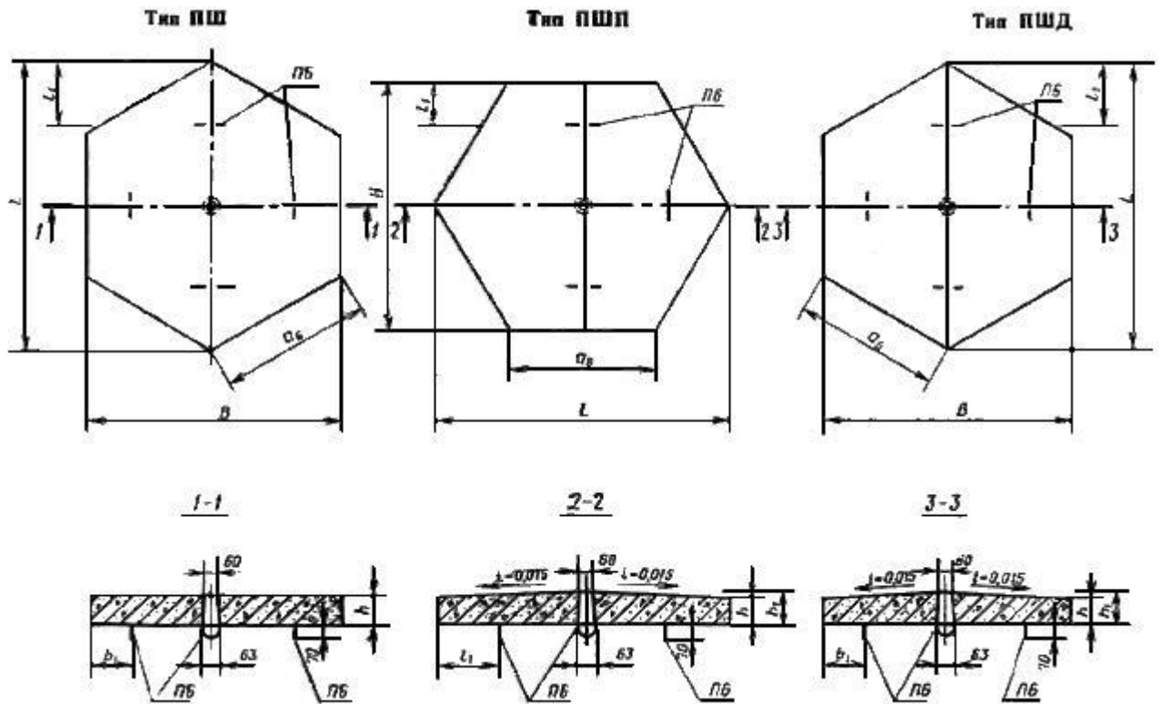
Черт.4. Форма и основные размеры плит. Типы ПШ, ПШП, ПШД
