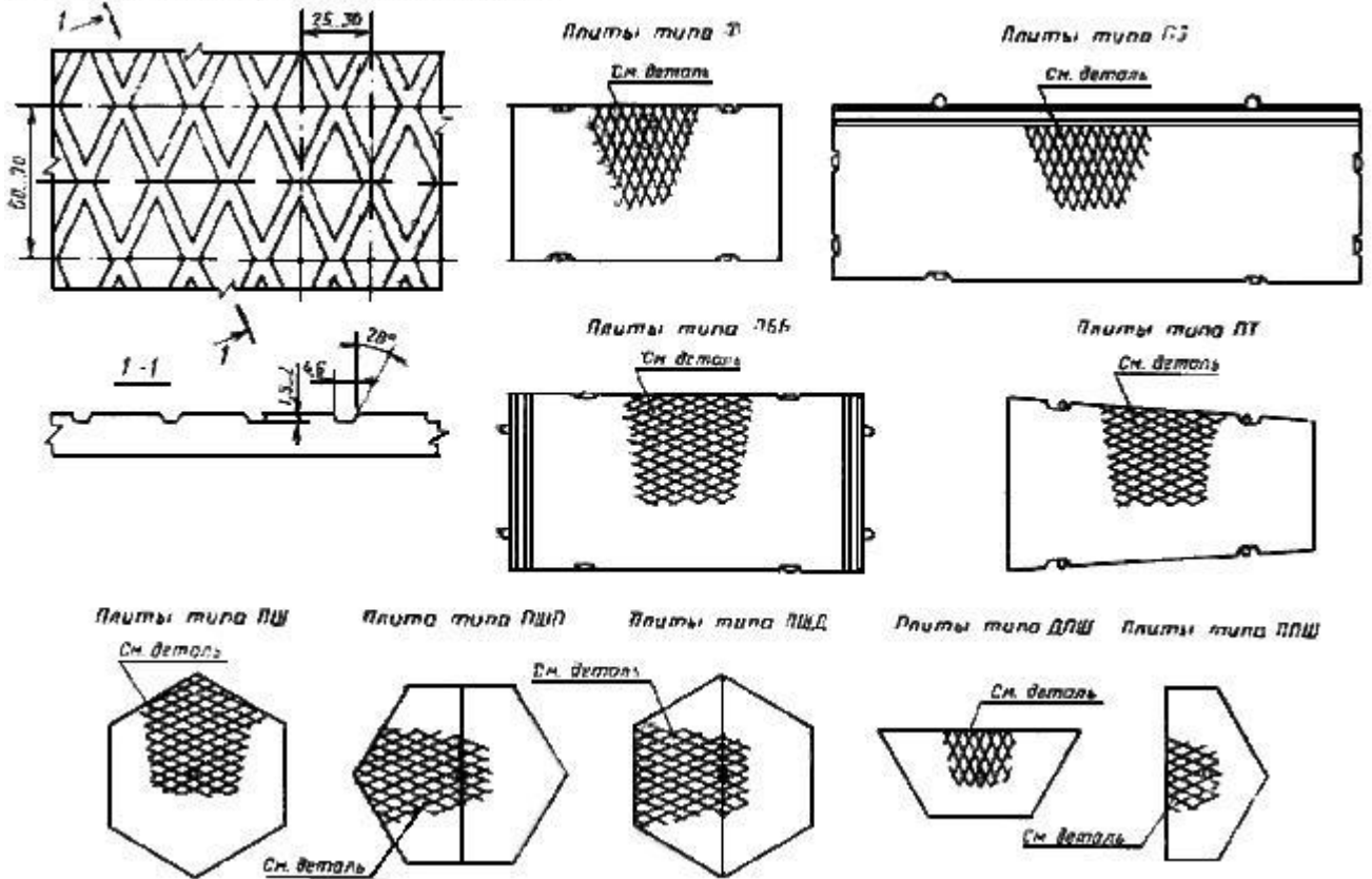
Деталь расфлеса на рабочей поверхности плиты
